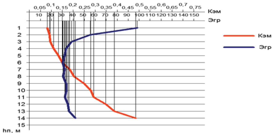
Рисунок 6. Зависимости эффективности свай по несущей способности по грунту и коэффициента использования материала сваи от глубины погружения (круглое сечение диаметром 0,45 м)
