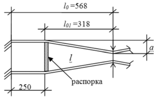
Рисунок 6. Расчетная схема затяжки по II-му варианту
