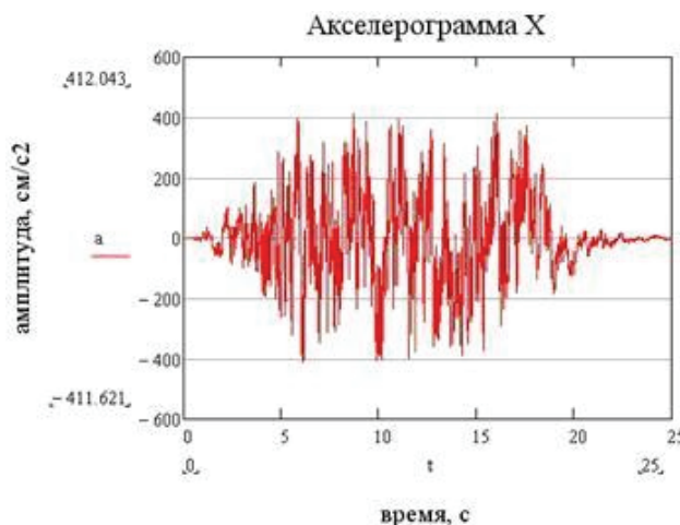
Рисунок 2. Синтезированная акселерограмма по направлению «X»
