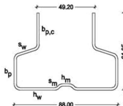
Рисунок 1. Поперечное сечение профиля
