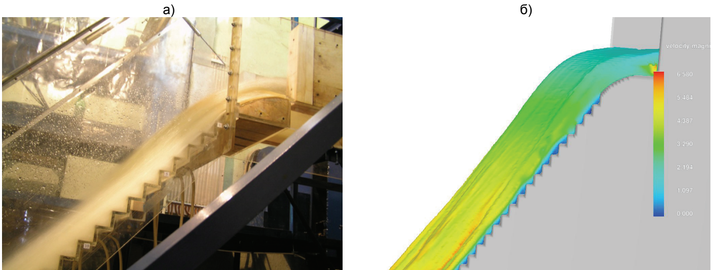
Рисунок 6. Вид на фрагмент струи на физической (а) и математической (б) моделях ступенчатого водосброса №2 Богучанского гидроузла (М1:30)
