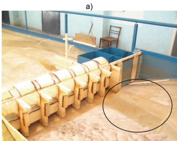
Рисунок 1. Вид с верхнего бьефа на физическую (а) и трехмерную компьютерную геометрическую (б) модели Нижне-Зейского гидроузла (М1:100). Черным обведены различия в построении моделей со стороны верхнего бьефа
