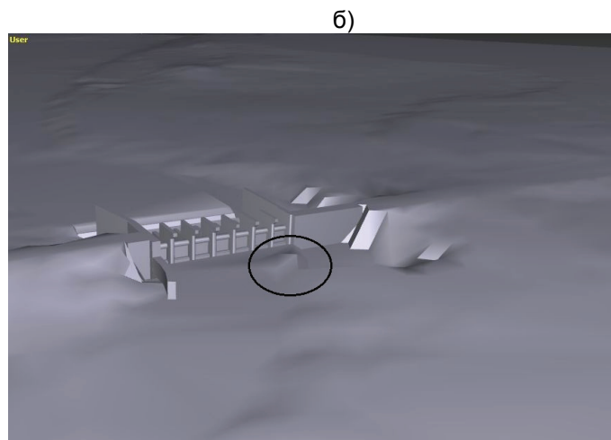
Рисунок 1. Вид с верхнего бьефа на физическую (а) и трехмерную компьютерную геометрическую (б) модели Нижне-Зейского гидроузла (М1:100). Черным обведены различия в построении моделей со стороны верхнего бьефа
