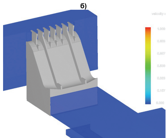
Рисунок 3. Вид с нижнего бьефа на физическую (а) [10] и трехмерную компьютерную геометрическую (б) модели водосброса Бурейского гидроузла (М1:100)
