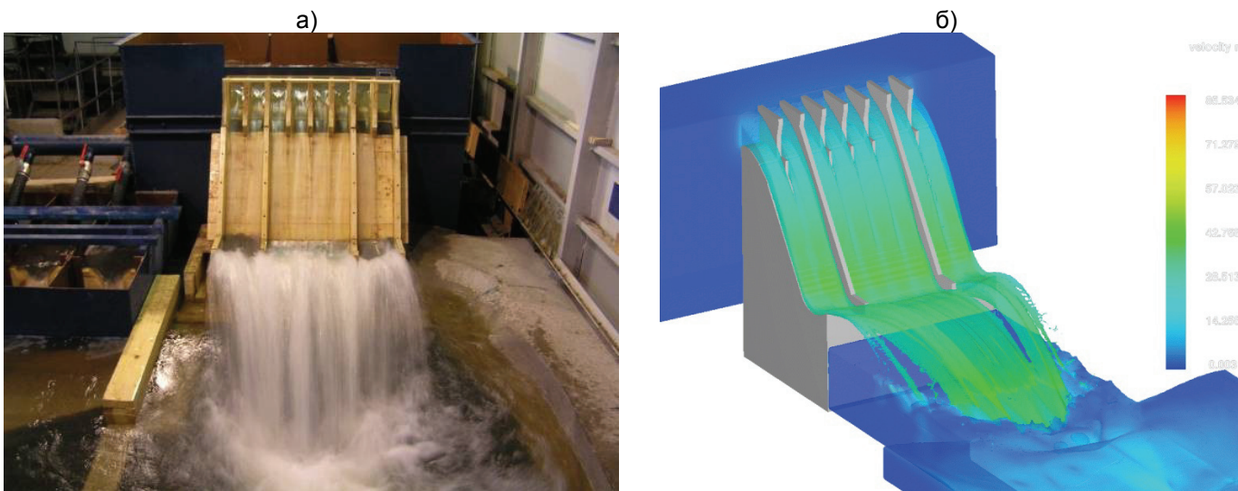
Рисунок 8. Вид на струю на физической (а) и математической (б) моделях водосброса Бурейского гидроузла (М1:100)
